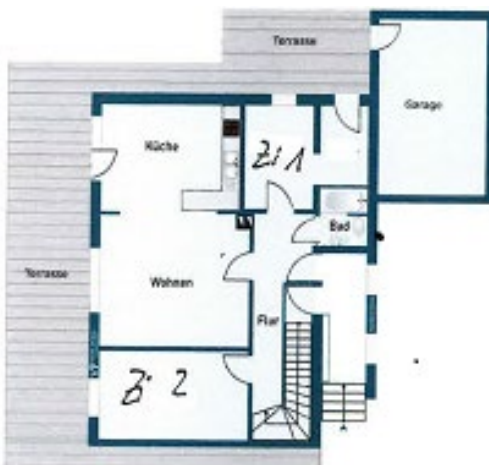
Grundriss EG
